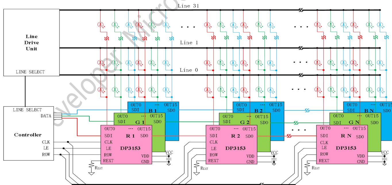
DP3153 典型应用原理图
