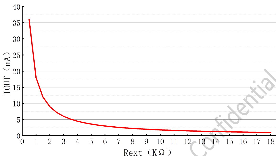
IGAIN=100%, R EXT 与 I OUT 之间的关系曲线
