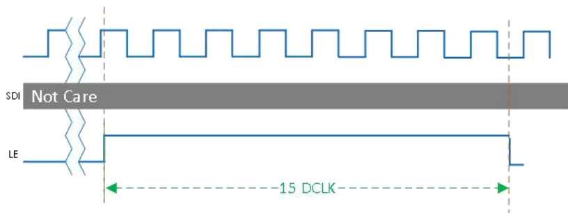
15 个 DCLK 边沿 (上升+下降) 设置为 SDR
