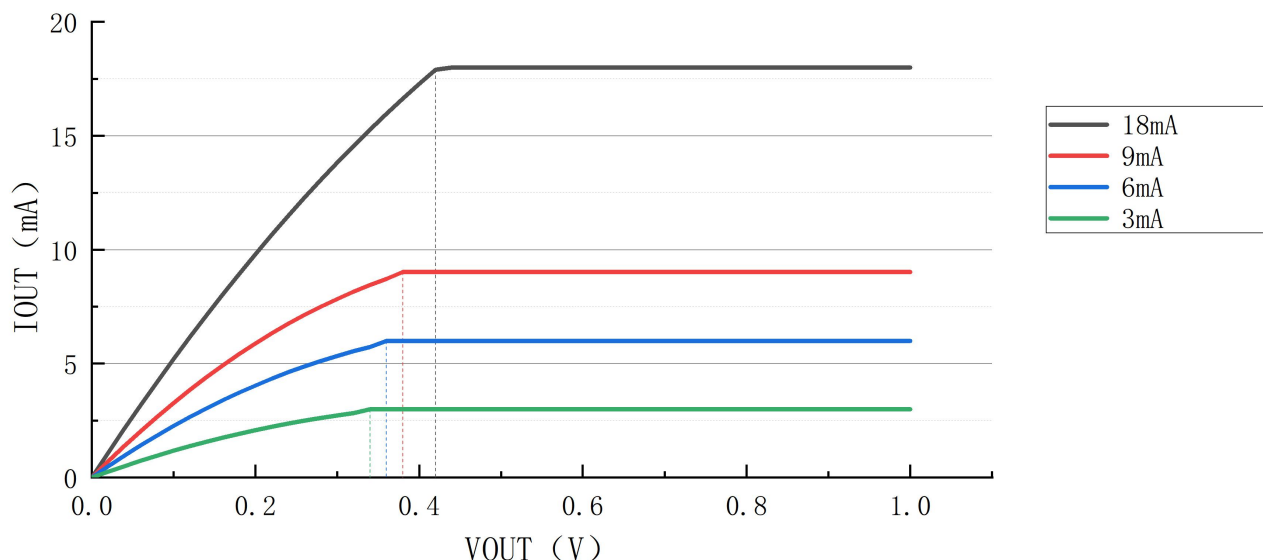
VDD=3.5V-5.5V 时，IOUT 与 VOUT 之间的关系曲线
