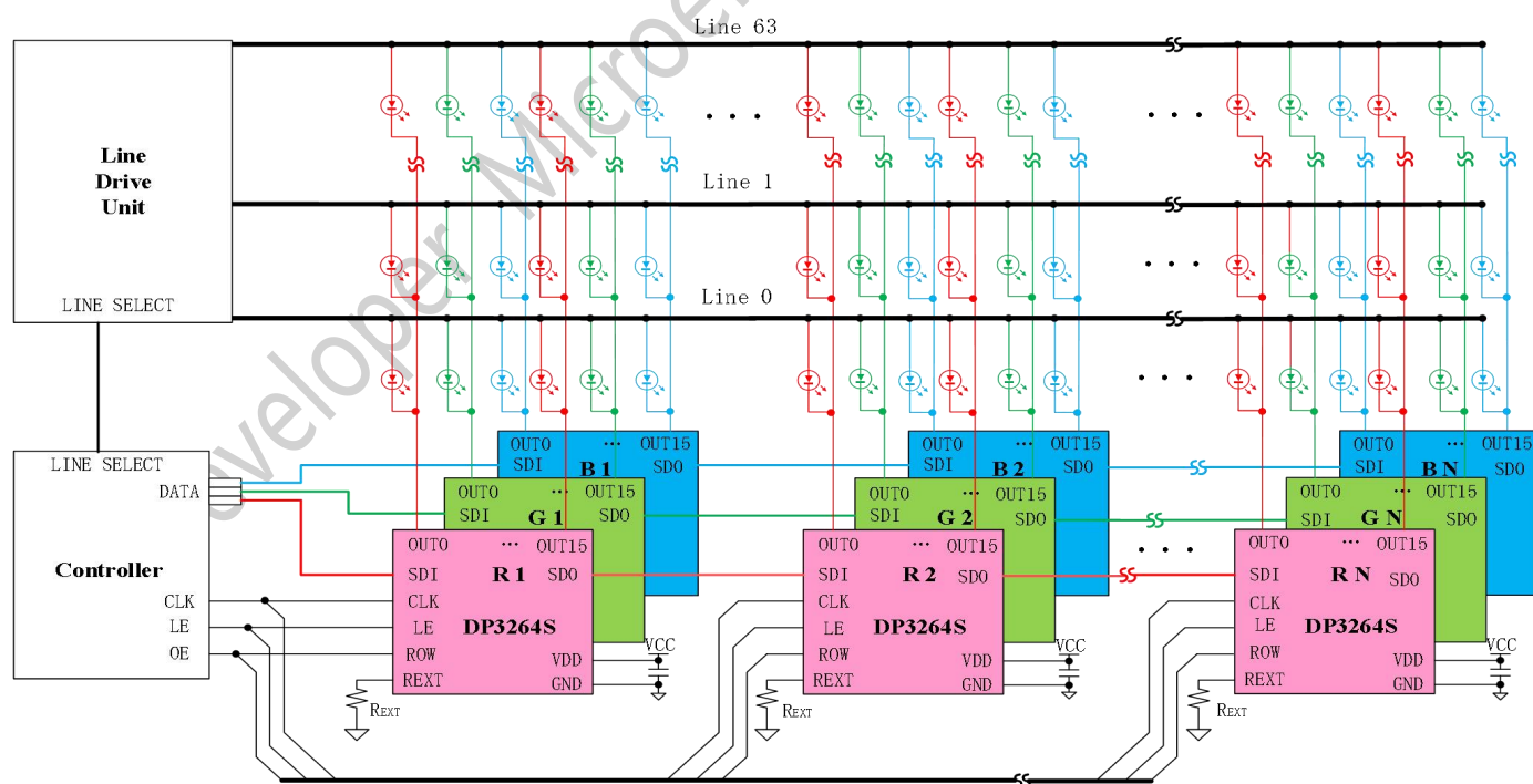
DP3264S 典型应用原理图
