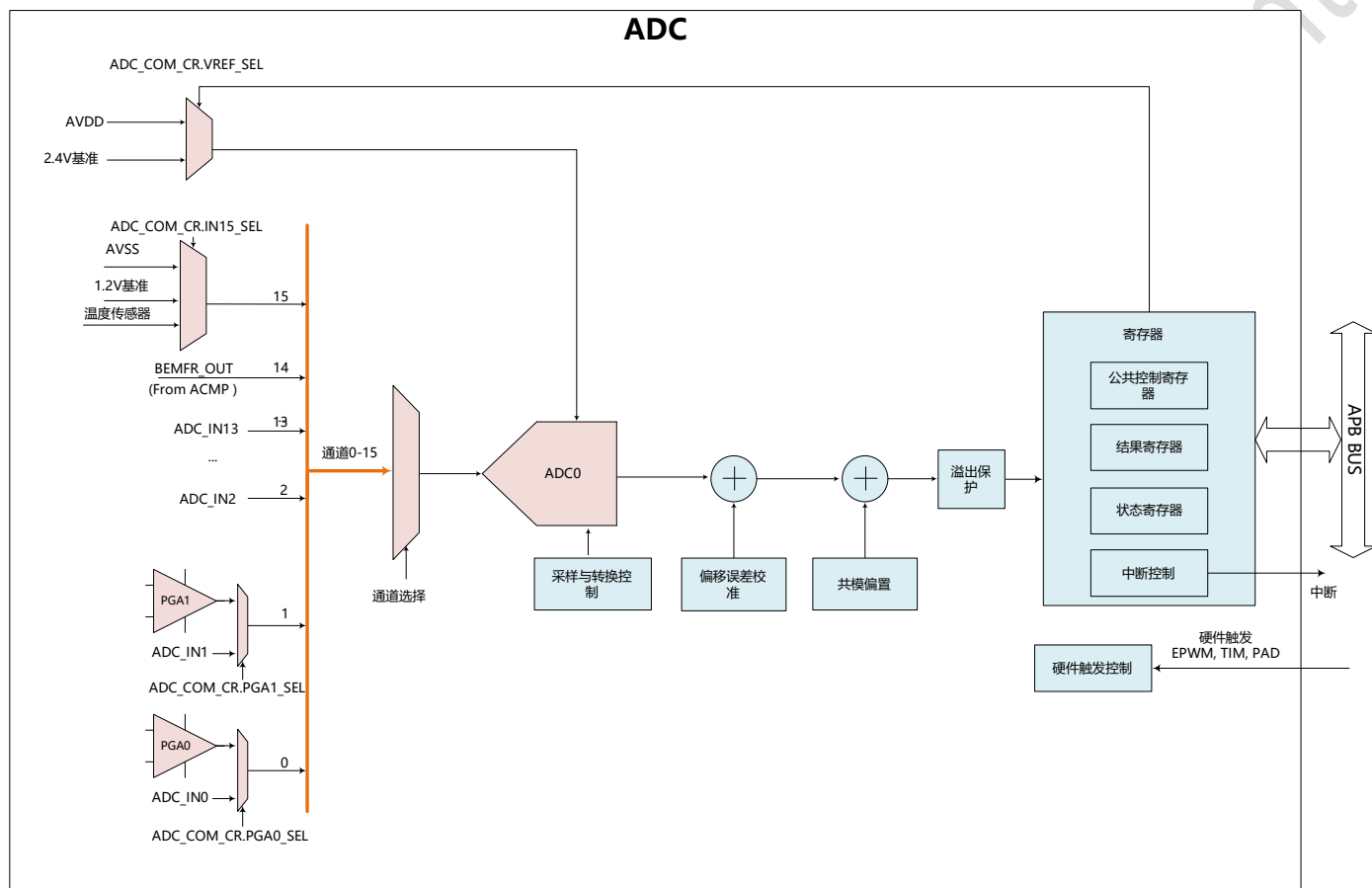
图 19-1 ADC 模块结构框图
