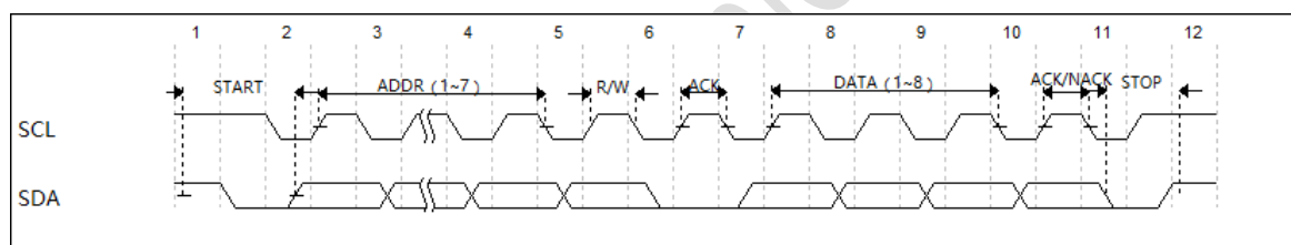
图 15-5 I2C 总线数据传输时序
