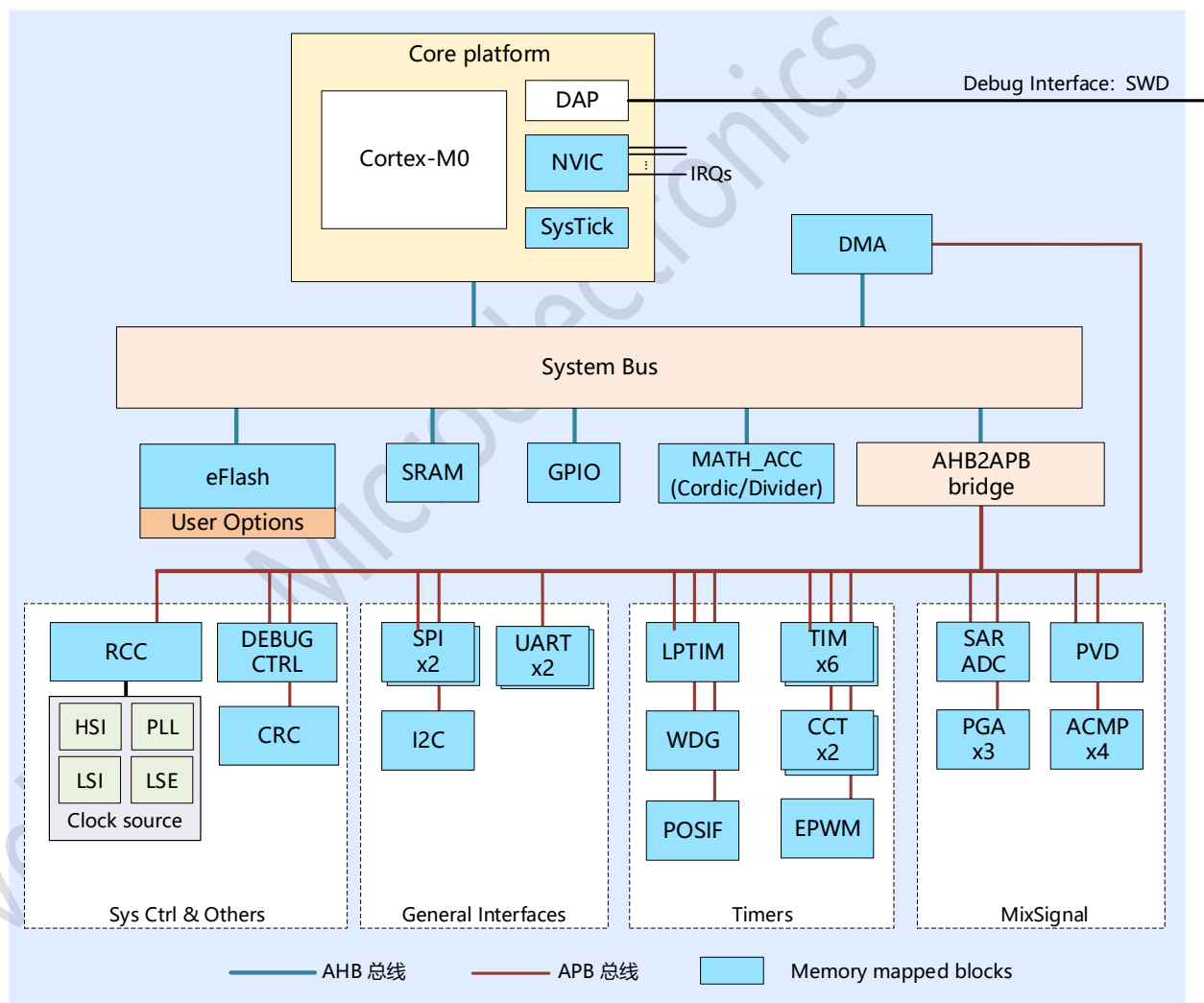
图 2-1 系统架构
