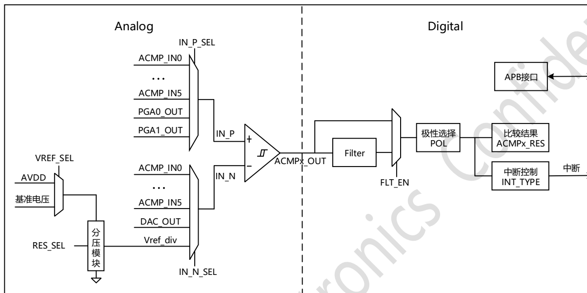
图 25-1 ACMPx 结构框图
