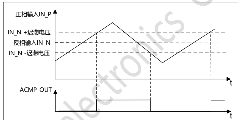
图 25-2 比较器迟滞
